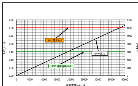
40K トルク特性
