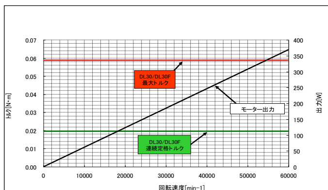
DL30/DL30F トルク特性
