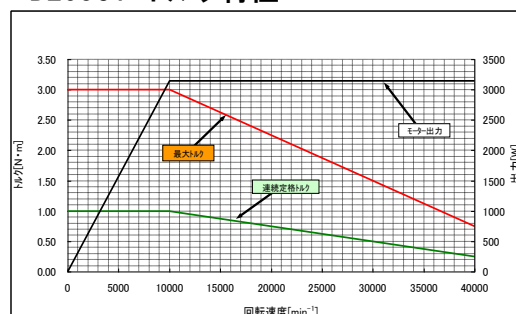
DL68CT トルク特性
