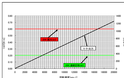
20K トルク特性
