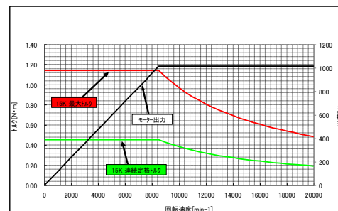
15K トルク特性
