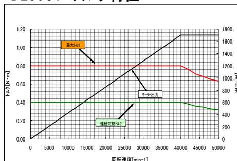
DL56CT トルク特性
