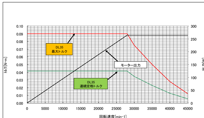
DL35 トルク特性
