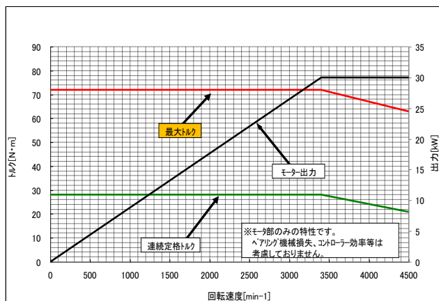
DL200 トルク特性
