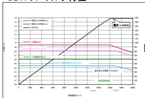
DL47CT トルク特性
